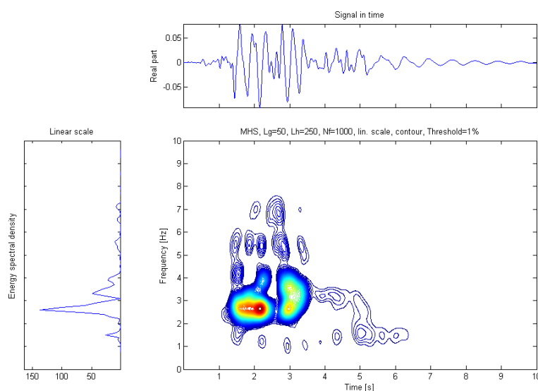
شکل ۷. تاریخچه زمانی شتاب‌نگاشت زلزله محاسبه شده در تاج در حالت پی صلب (تصویر بالا)، چگالی طیفی انرژی (تصویر سمت چپ) و تبدیل حوزه زمان - فرکانس نگاشت مذکور (تصویر سمت راست)
