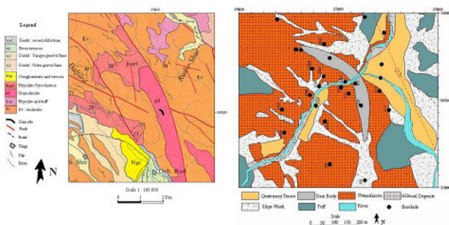
شکل ۱. نقشه زمین‌شناسی محدوده ساخت‌گاه سد شور- چیرفت و موقعیت گمانه‌های اکتشافی [۱]
