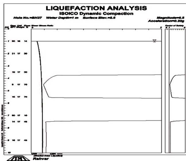
شکل ۱۲. نتیجه تحلیل روان‌گرایی گمانه Z4-BH27 با فرض وقوع زلزله به شتاب g/200 و بزرگی 6/5 [۱]
