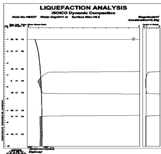
شکل ۱۱. نتیجه تحلیل روان‌گرایی گمانه Z4-BH27 با فرض وقوع زلزله به شتاب g/250 و بزرگی 7/0 [۱]
