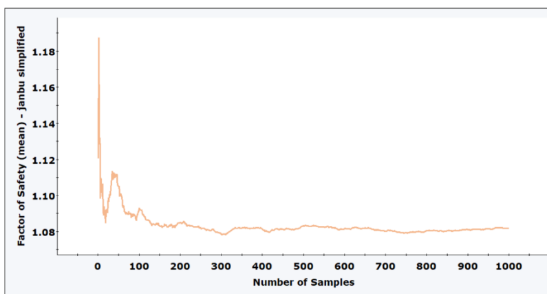
شکل ۱. همگرایی نتایج آنالیز احتمالاتی برای ۱۰۰۰ نمونه
