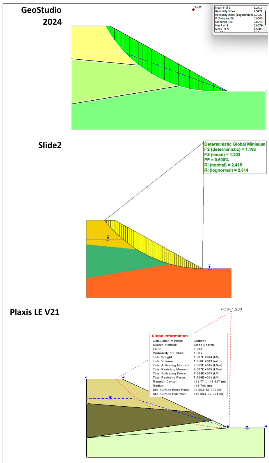
شکل ۵. نتایج آنالیز احتمالاتی پایداری شیب در حالت خاک لایه ای در سه نرم افزار (روش سپاه مهندسين ۱، بعنوان نمونه)
