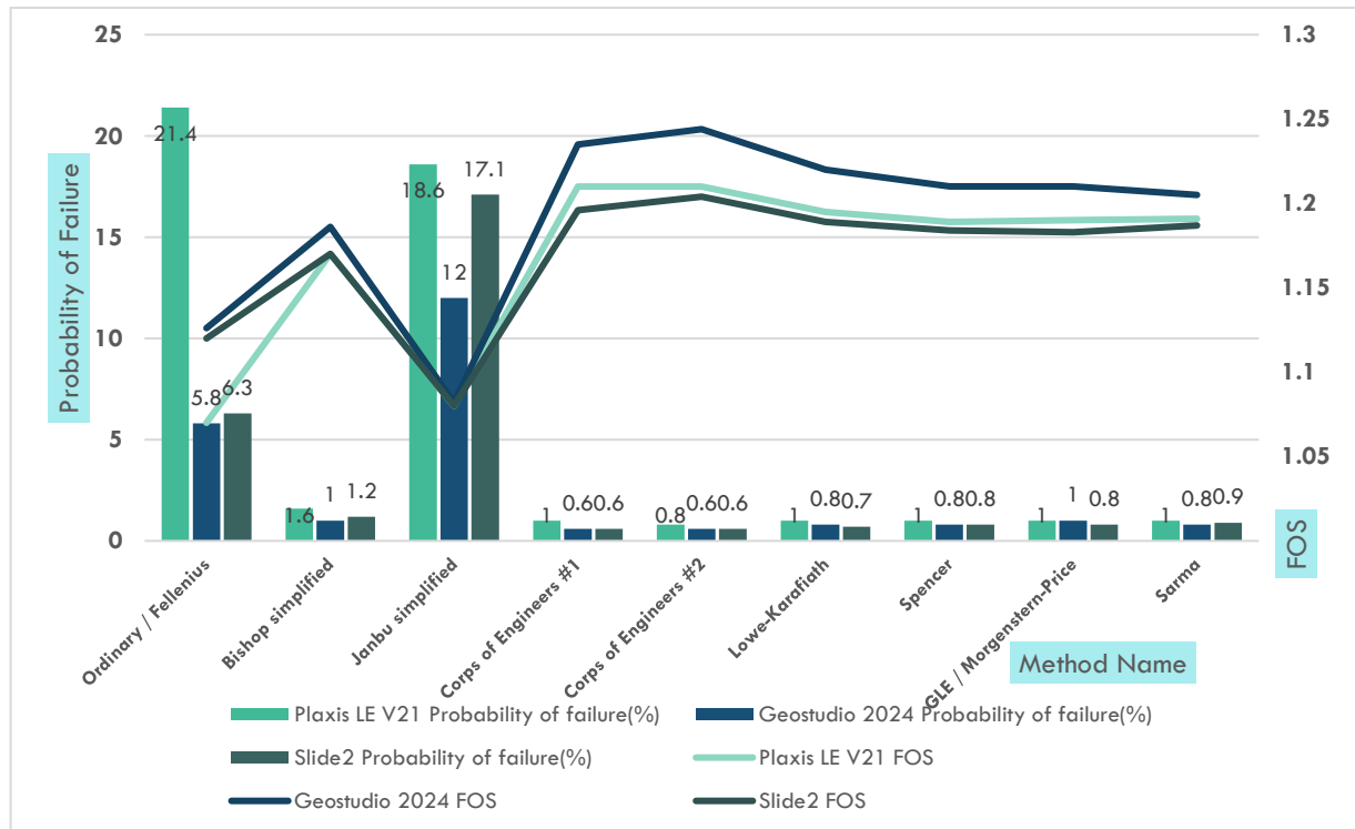
شکل ۶. نتایج کامل آنالیز احتمالاتی پایداری شیب در حالت خاک لایه‌ای در سه نرم‌افزار Fig. 6. Full results of probabilistic analysis of slope stability in layered soil condition in three software
