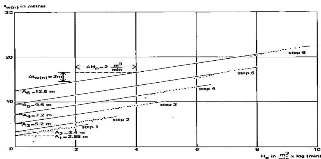
شکل ۴. روش ایدن - هیزل، داده‌های (sW(n)) در برابر مقادیر H_n (Kruselman and de Ridder, 1994)
