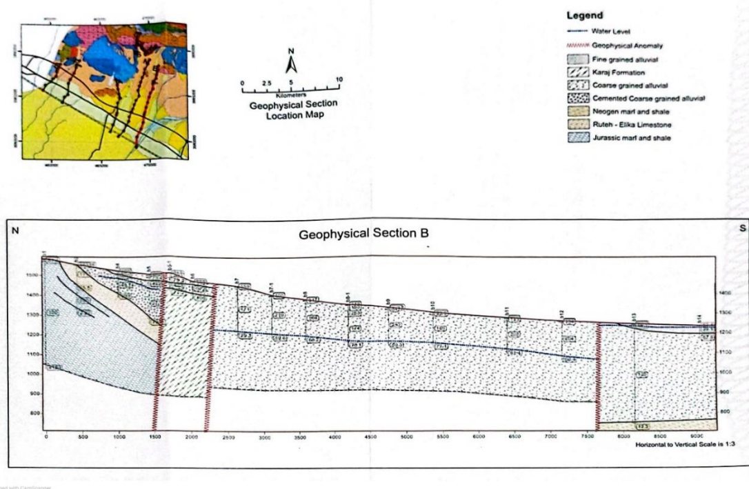
شکل ۱۲. مقطع ژئوفیزیک B
