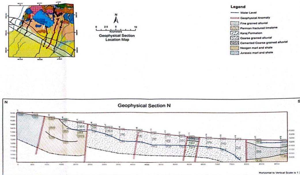
شکل ۱۱. مقطع ژئوفیزیک N
