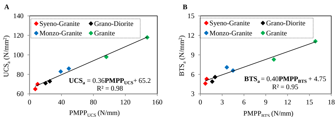
شکل ۱۴. رابطه دوام سنگ در برابر انجماد و آب شدن با پارامتر پترو-مکانیکی (A) مقاومت فشاری تک محوری (B) مقاومت کششی برزیلین نکته: دوام سنگ از طریق مقادیر مقاومت فشاری تک محوری (UCS a ) و مقاومت کششی برزیلین (BTS a ) بعد از فرایندهای انجماد و آب شدن ارزیابی شده است
