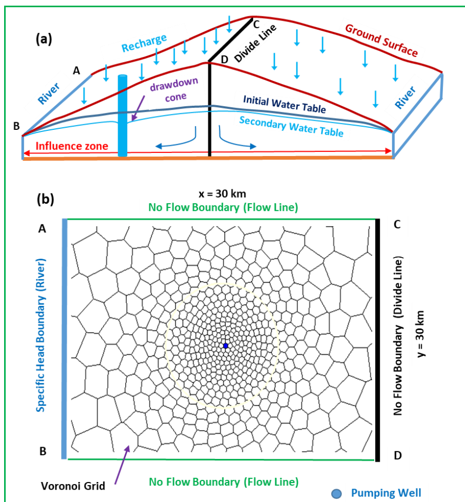
شکل ۱. مدل مفهومی، شرایط مرزی و شبکه‌بندی استفاده شده در مادفلو برای شبیه‌سازی چاهی در مرکز آبخوان.
