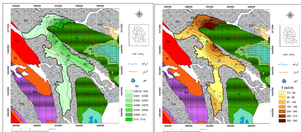
شکل ۵. نقشه پهنه بندی قابلیت انتقال (سمت راست) پهنه بندی آبدهی ویژه (سمت چپ) بر اساس روش دانه بندی
