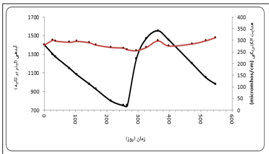
شکل ۹- تغییرات زمانی هدایت الکتریکی و دبی چشمه کارستنی ورسخواران
