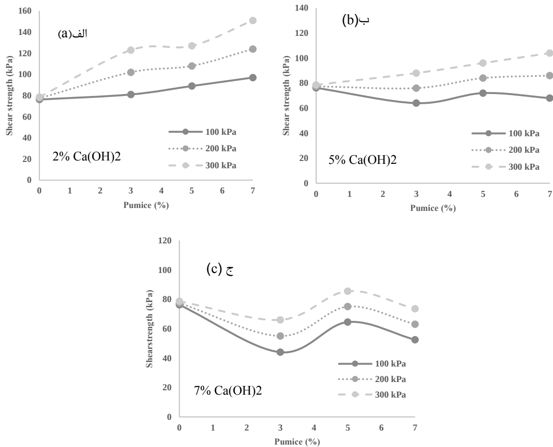
شکل ۹. تأثیر ترکیب پومیس و هیدروکسید کلسیم بر روی مقاومت برشی نمونه‌های مورد مطالعه، الف- ۲٪ هیدروکسید کلسیم، ب- ۵٪ هیدروکسید کلسیم، ج- ۷٪ هیدروکسید کلسیم.
