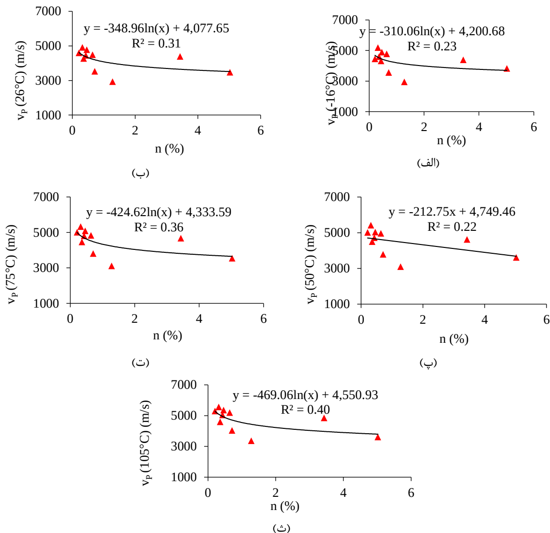
شکل ۴. ارتباط بین تخلخل و سرعت موج التراسونیک سنگ‌های مورد مطالعه در دماهای (الف) -16^\circ\text{C} ، (ب) 26^\circ\text{C} ، (پ) 50^\circ\text{C} ، (ت) 75^\circ\text{C} و (ث) 105^\circ\text{C} درجه سانتی‌گراد
