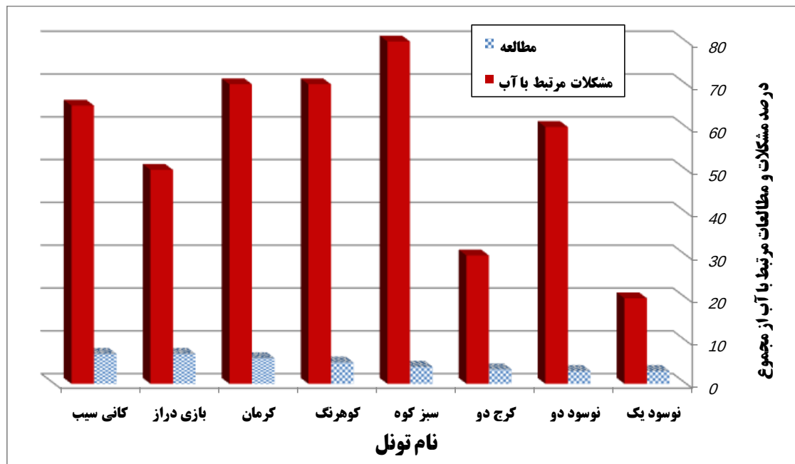
شکل ۳. نسبت مطالعات هیدروژئولوژی و مشکلات مرتبط با هیدروژئولوژی در پروژه‌های تونلی Fig. 3. Comparison of hydrogeology studies and problems related to hydrogeology in tunnel projects
