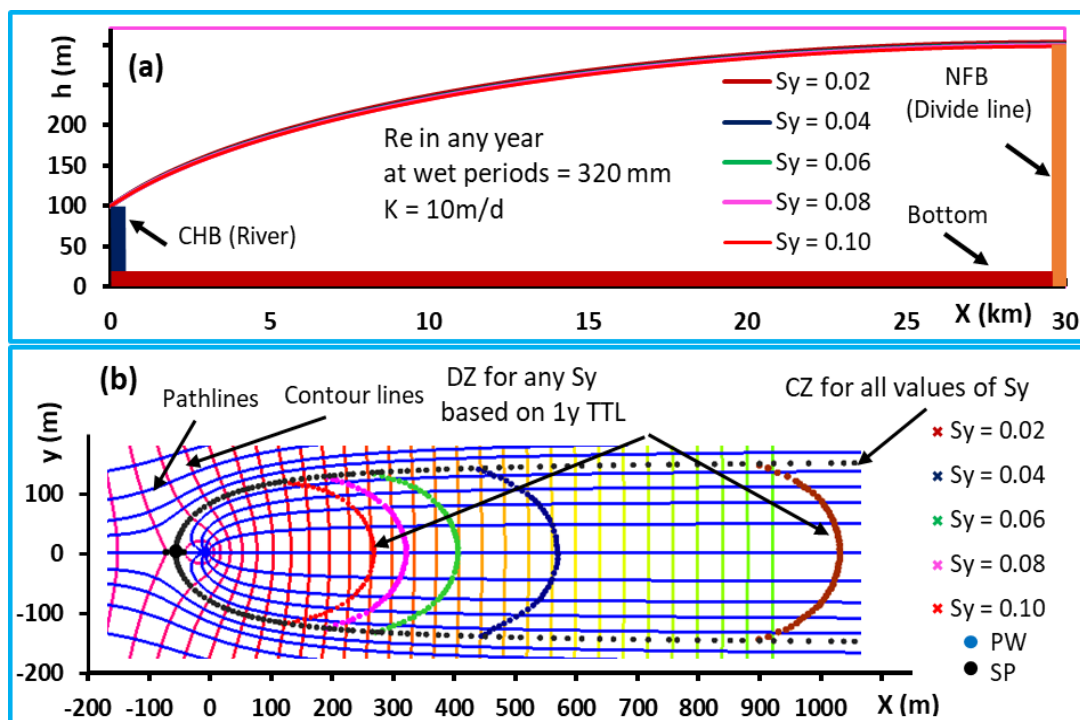
شکل ۶. اثر آبدهی ویژه ( S_y ): (a) سطح آب نرمال در پایان دوره‌ی تر. (b) حریم آبرگیر و حریم تخلیه. خطوط زمان گذر یک ساله هستند.
