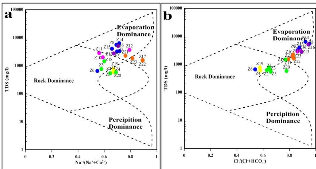
شکل ۵. نمودار گیبس نمونه‌های آب زیرزمینی
