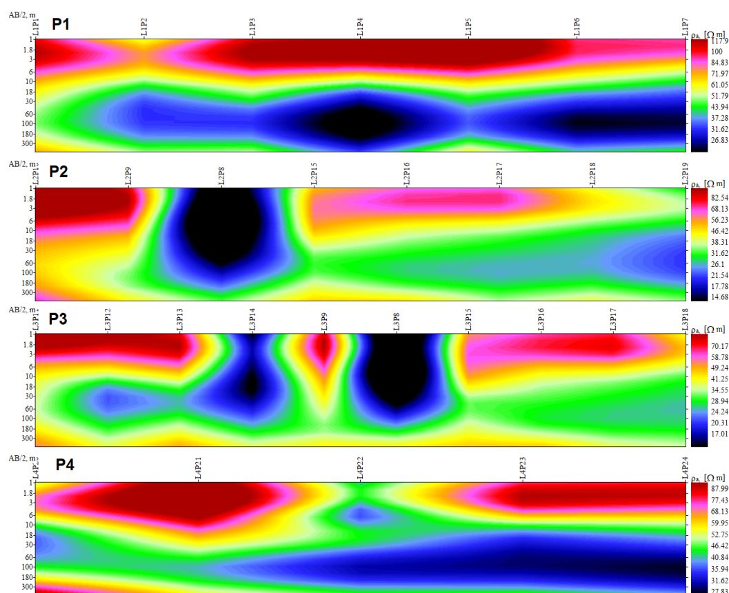
شکل ۷. شبه مقطع ژئوالکتریکی در پروفیل اول تا چهارم Fig.7. Goelectric quasi-section in the first to fourth profiles
