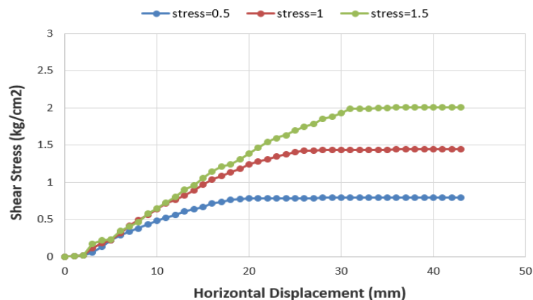
شکل ۱۴- نمودار جابجایی بر حسب تنش برشی میانگین نمونه شماره ۵، ۶، ۷، ۸ و ۹ همراه با ضایعات کم
