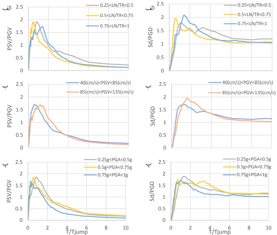
شکل ۷- طیف پاسخ جابجایی نرمال دوسویه با معیار گام T_{jump} (با نماد BNDS(T_{jump}) ) شکل ۸- طیف پاسخ شبه سرعت نرمال دوسویه با معیار گام T_{jump} (با نماد BNPVS(T_{jump}) )
