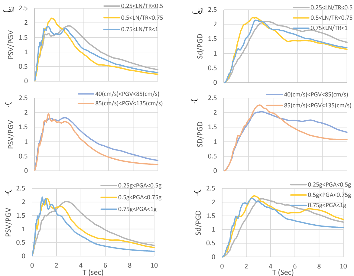
شکل ۳- طیف پاسخ جابجایی نرمال، (با نماد NDS)
