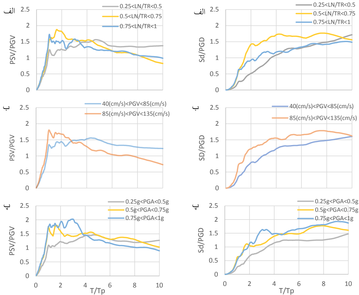
شکل ۵- طیف پاسخ جابجایی نرمال دوسویه با معیار پریود غالب T_p ، (با نماد (BNDS(T_p))
