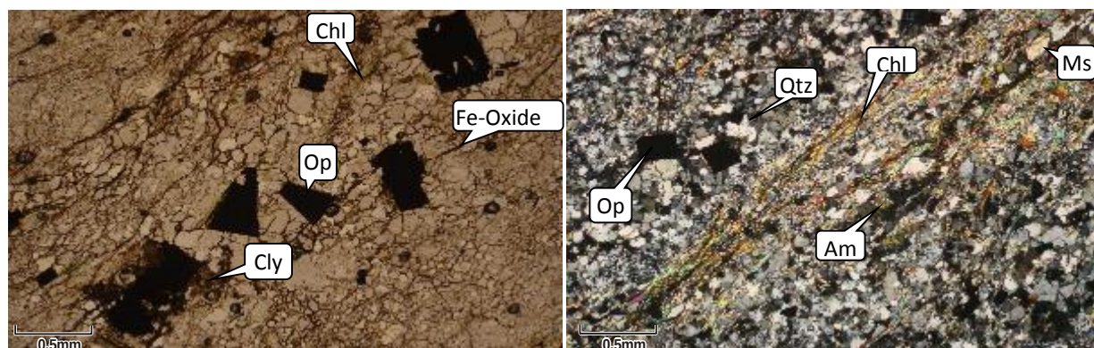
شکل شماره ۵ - مقطع کانی‌شناسی شیست (B2) - قرارگیری کانی‌های موسکوویت، یوتیت، کلریت در بین کانی‌های کوارتز و ایجاد فابریک شیستوزیته در نمونه (نور عبوری XPL). (سمت راست)؛ اکسید و هیدرواکسیدهای آهن به صورت آغشتگی و رگه-رگچه‌ای در نمونه مشاهده می‌شود (تصویر بالا در نور عبوری PPL). (سمت چپ).
