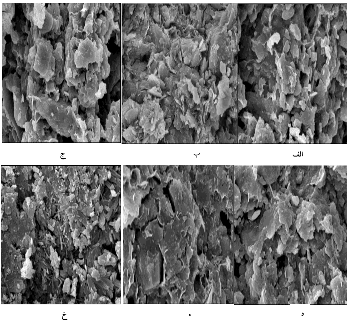
شکل ۶- نتایج SEM با بزرگ‌نمایی ۳۰۰۰ برابر، الف) خاک طبیعی، ب) خاک آلوده به ۴٪ محلول گلیسرول، ج) خاک آلوده به ۱۲٪ محلول گلیسرول، د) خاک طبیعی + ۱۲٪ MgO ، ه) خاک آلوده به ۴٪ محلول گلیسرول + ۱۲٪ MgO (۱۴روزه)، خ) خاک آلوده به ۱۲٪ محلول گلیسرول + ۱۲٪ MgO (۱۴روزه)
