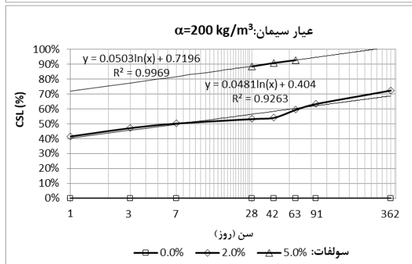
شکل ۸. تأثیر تغییر عیار سیمان و درصد سولفات بر پارامتر CSL برای نمونه‌های با سولفات ۲٪ و ۵٪ در الف) عیار (\text{kg/m}^3) ۴۰۰، ب) عیار (\text{kg/m}^3) ۳۰۰، ج) عیار (\text{kg/m}^3) ۲۰۰
