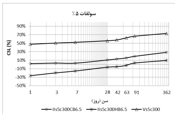
شکل ۱۲. تغییرات CSL مقاومت فشاری تک محوری در مقابل زمان برای سیمان تیپ ۵ و سیمان تیپ ۲ با عیار 300 \text{ (kg/m}^3\text{)} در ترکیب با کلرید باریم و هیدروکسید باریم در شرایط سولفات ۵٪
