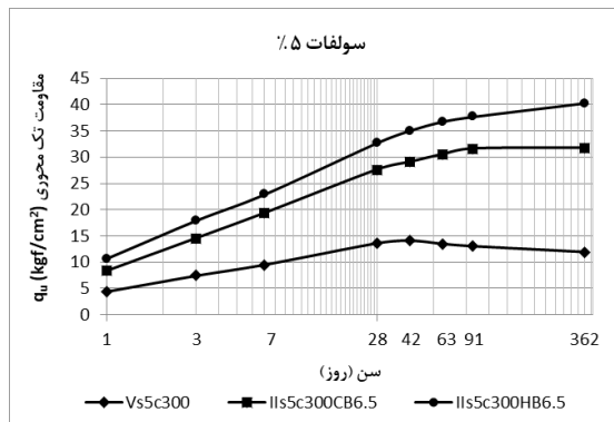
شکل ۱۱. تغییرات مقاومت فشاری تک محوری در مقابل زمان برای سیمان تیپ ۵ و سیمان تیپ ۲ در ترکیب با کلرید باریم و هیدروکسید باریم در شرایط سولفات ۵٪
