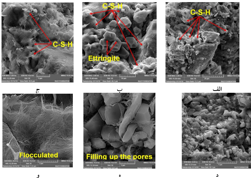
شکل ۶. ریزساختارهای نمونه خاک شماره دو (MCS)
