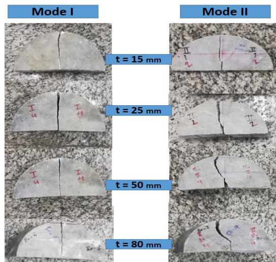
شکل ۶. نمونه‌های SCB مرمریت پس از آزمایش شکست. جدول ۲. بار شکست نمونه‌های SCB با ضخامت‌های مختلف
