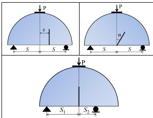
شکل ۲. حالت‌های مربوط به بارگذاری مود ترکیبی I/II جدول ۱. اندازه قطعات آزمایش و شرایط بارگذاری مربوط
