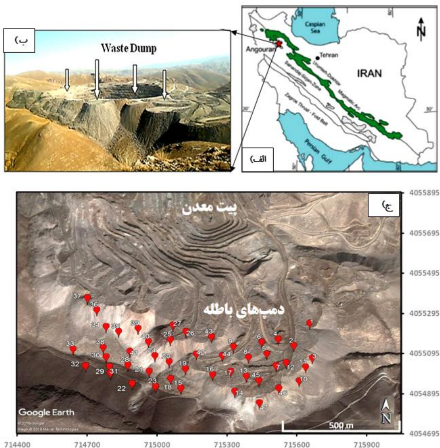
شکل ۳. الف) موقعیت معدن سرب و روی انگوران در شمال غربی زون سنندج-سیرجان [۲۴]، ب) نمایی از قرارگیری دب‌های باطله در جنوب پیت معدن، ج) موقعیت جغرافیایی نمونه‌های برداشت شده از محدوده بررسی شده [عکس گرفته شده از Google Earth]
