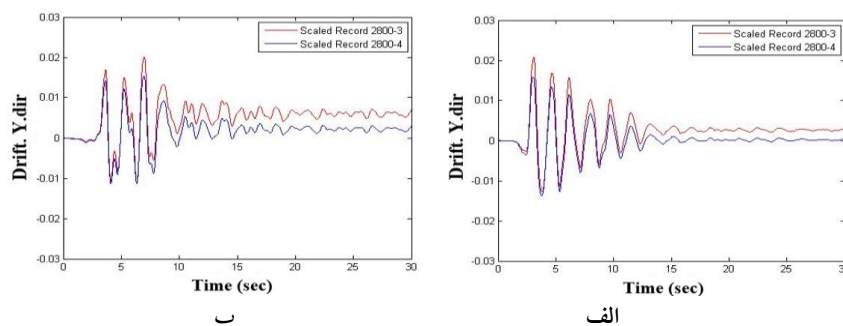
شکل ۱۷. تاریخچه زمانی دررفت طبقه بام مدل ۱۰ طبقه تحت اثر دو رکورد، الف) رکورد ۳، ب) رکورد ۴ SCE
