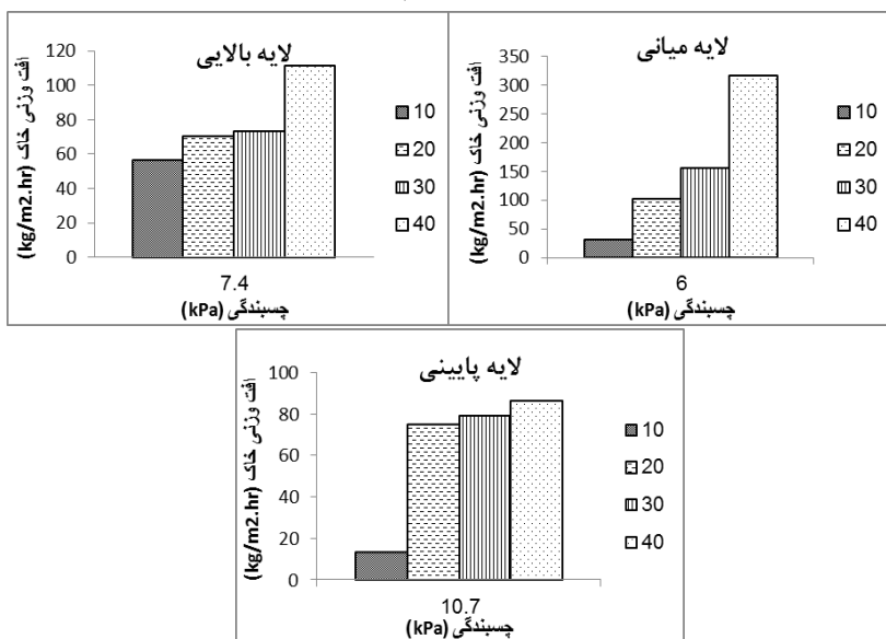
شکل ۲۰. رابطه کسبندگی با فرسایش پذیری سه لایه خاک
