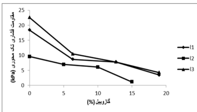
شکل ۹. تغییرات مقاومت فشاری تک محوری در مقابل گازوییل
