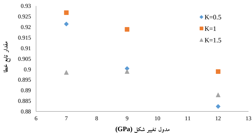
شکل ۶. تغییرات تابع خطا در مقابل مدول تغییر شکل، الف) رابطه ۱، ب) رابطه ۲
