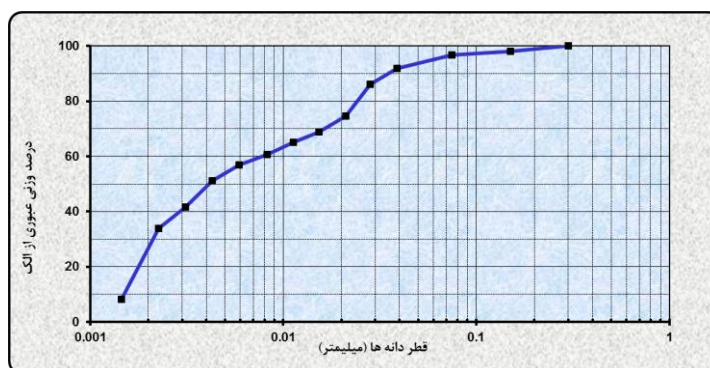
شکل ۱. منحنی دانه‌بندی خاک استفاده شده
