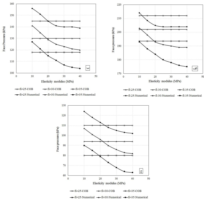
شکل ۷. مدول الاستیسیتة- فشار جبهه کار برای تراز آب الف (۰، ب ۹، ج ۲۷ متری از سطح زمین)
