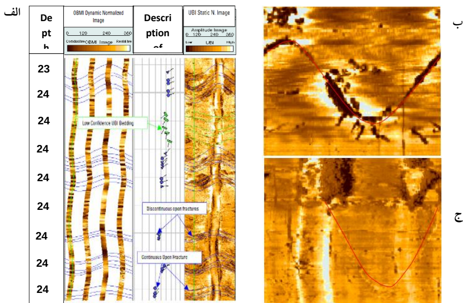
شکل ۶. الف) پردازش نگاره‌های تصویری OBMI و UBI در چاه C، ب و ج) به ترتیب شکستگی‌های باز و بسته
