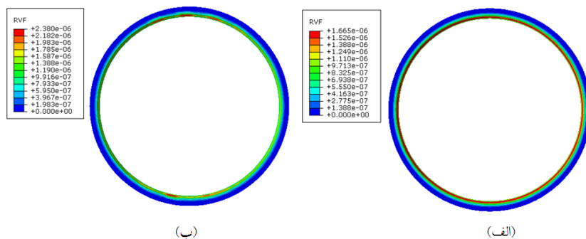
شکل ۶. مقایسه دبی نشست آب از تونل در دو توزیع میلگرد؛ الف) ۲۰ cm @ \Phi 16 mm و ب) ۳۰ cm @ \Phi 20 mm
