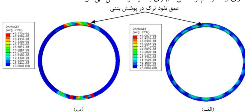
شکل ۷. مقایسه تعداد و عمق ترک‌ها در دو توزیع میلگرد: الف) 20\text{ cm} @ \Phi 16\text{ mm} و ب) 30\text{ cm} @ \Phi 20\text{ mm}
