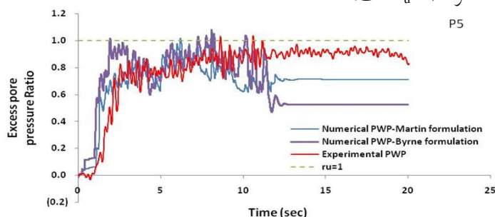
شکل ۱۱. مقایسه تاریخچه نسبت فشار آب حفره‌ای مدل‌سازی عددی و آزمایش ساتریفوژ در عمق ۱/۴۵ متر
