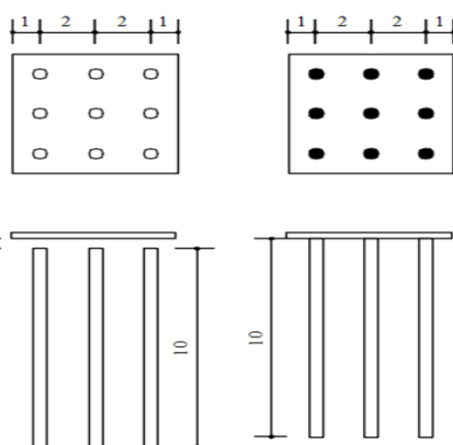
شکل ۵. نمای پلان و کنار ابعاد و محل اتصال پی رادیه-شمع متصل (سمت راست) و منفصل (سمت چپ) (واحد: متر)
