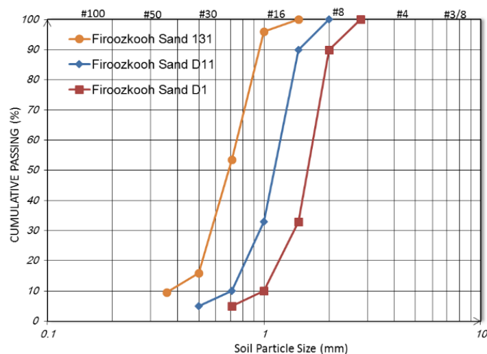
شکل ۱. نمودار دانه‌بندی ماسه‌های استفاده شده
