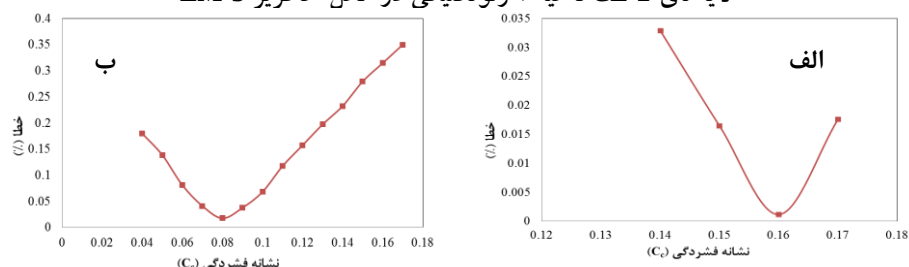
شکل ۲۰. الف) نمودار کمیته‌سازی تابع خطا برای پارامتر نشانه فشردگی ( C_c ) در لایه ML ناحیه ۲ ژئوتکنیکی، ب) نمودار کمیته‌سازی تابع خطا برای پارامتر نشانه فشردگی ( C_c ) در لایه CL-1 ناحیه ۲ ژئوتکنیکی
