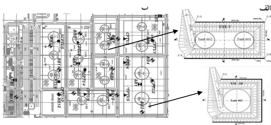
شکل ۷. الف) پلان موقعیت خاکریزهای EM-3 و EM-2B، ب) محل گمانه های ناحیه دو و سه ژئوتکنیکی
