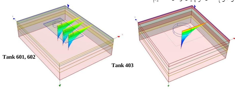
شکل ۲۴. مدل‌سازی مخازن Tank 403 و Tank 601 و Tank 602 در برنامه Settle 3D
