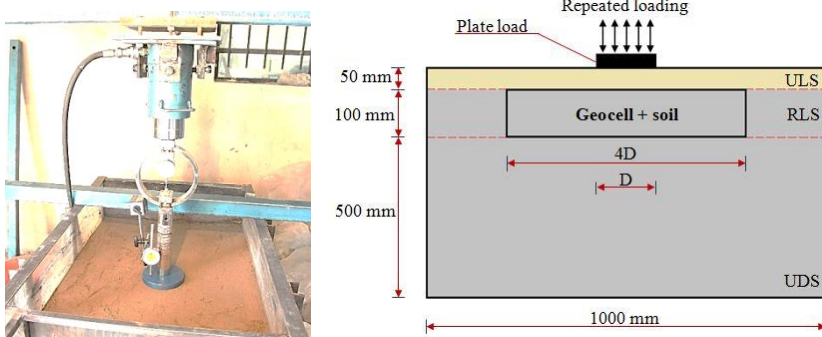
داس و عمر ۱ در سال ۱۹۹۴ اعلام کردند که ظرفیت باربری بستر مسلح و غیرمسلح برای صفحه‌های بارگذاری با قطر بیش از ۱۵۰ میلی‌متر تغییرات چندانی ندارد و انتخاب صفحه دایره‌ای به قطر ۱۵۰ میلی‌متر کفایت می‌کند [۲۸]. هم‌چنین هسی و مائو ۲ در سال ۲۰۰۵ با بارگذاری روی خاک با دو صفحه دایره‌ای به قطرهای ۱۵ و ۳۰ سانتی‌متر و دانه‌بندی مختلف دریافتند که صفحه بارگذاری با اندازه بزرگ‌تر از ۱۵ برابر اندازه D ۵۰ خاک تأثیر چندانی بر نشست صفحه ندارد [۲۹]. در این پژوهش D ۵۰ برابر با ۰/۲۱۹ میلی‌متر است. آرنولد در سال ۲۰۰۴ به‌منظور بررسی شیار افتادگی چرخ کامیون سنگین از بار ۱۰۰۰ کیلو پاسکال استفاده کرده است [۳۰]. توکلی و همکاران نیز در سال‌های ۲۰۱۳ و ۲۰۱۵ برای شبیه‌سازی اثر چرخ خودرو با تنش حداکثر ۸۰۰ کیلوپاسکال از صفحه بارگذاری دایره‌ای شکل به قطر ۱۵۰ میلی‌متر برای این منظور استفاده کردند [۲۳]، [۳۱]. خلیج و همکاران در سال ۲۰۱۵ به‌منظور مدل کردن بار کامیون سنگین در حالت پر از بار و کامیون بدون بار، به‌ترتیب نیروی ۸۰۰ و ۴۰۰ کیلو پاسکال را انتخاب کرده‌اند [۳۲]. در پژوهش حاضر به‌منظور مدل‌سازی بار وسایل نقلیه سبک نظیر وانت، نیروی ۲۵۰ کیلو پاسکال در سطح اول بارگذاری، نیروی ۵۰۰ برای کامیون نیمه‌پر، نیروی ۷۵۰ برای کامیون پر از بار و نیروی ۱۰۰۰ کیلو پاسکال برای تعیین حداکثر بار قابل تحمل انتخاب شده است.
