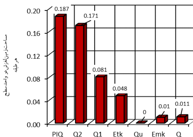
واحدهای لیتولوژی
