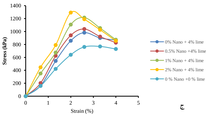
شکل ۳. مقاومت تک‌محوری خاک همراه با درصد‌های مختلف افزودنی آهک و نانورس (الف) نمونه‌ها بدون افزودنی آهک (ب) نمونه‌ها با ۲ درصد آهک (ج) نمونه‌ها با ۴ درصد آهک
