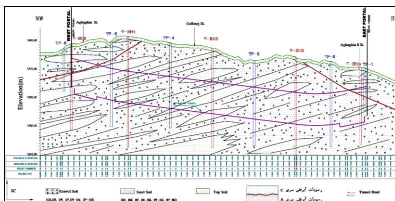
شکل ۵. پروفیل زمین‌شناسی و موقعیت گمانه‌های حفاری شده در مسیر تونل حکیم
