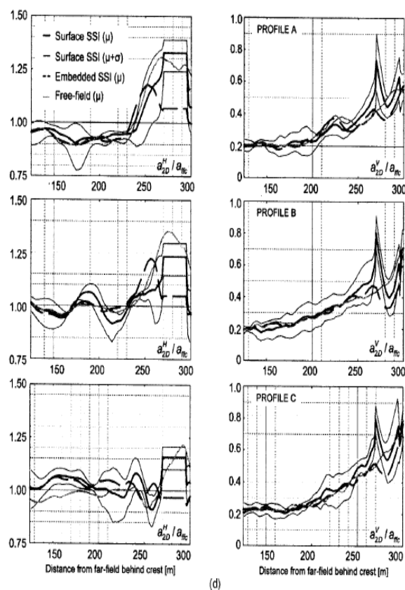
شکل ۳. تأثیر حضور سازه بر تغییر پاسخ شتاب در مجاورت توپوگرافی شیب در سه پروفیل خاک تحت آنالیز غیرخطی [۸]
