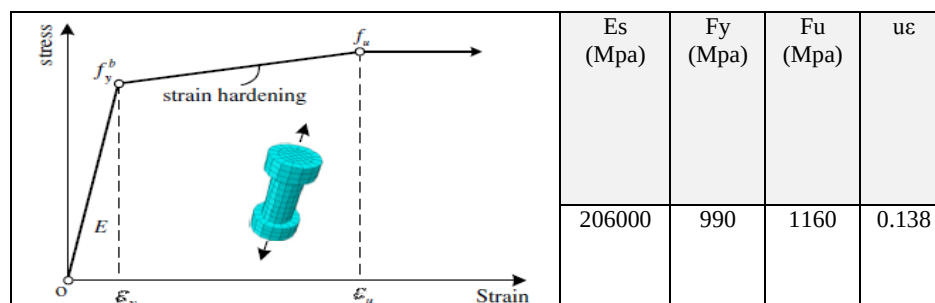
شکل ۱۳. مدل رفتاری پیچ پرمقاومت
