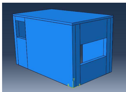
شکل ۴. ساختمان شماره ۳ مدل شده در نرم‌افزار ABAQUS ، الف) نمای پنجره‌هایی بزرگ و نزدیک به لبه دیوار، ب) نمای دیوار با بازشو ورودی
