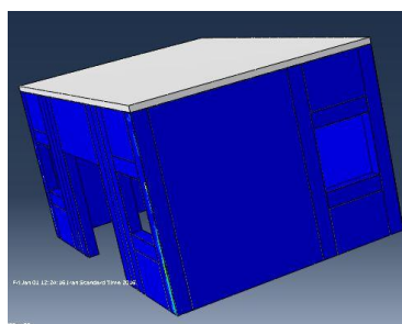
شکل ۱۷. کانتور کرنش‌های پلاستیک اصلی پیشینه بعد از تقویت در مقابل زلزله طبرس که در ایستگاه کاشمر (خاک نوع III) ثبت شده است
