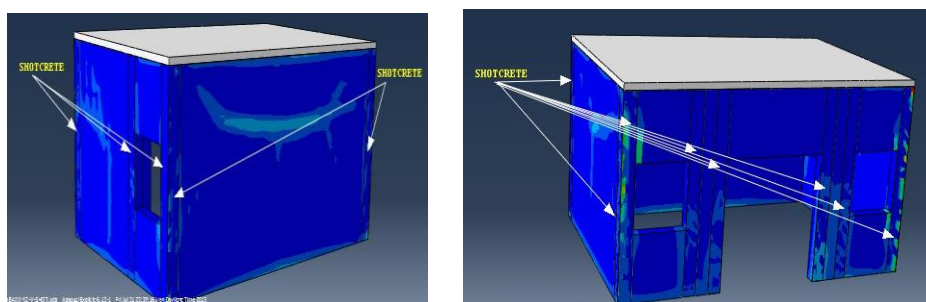
شکل ۱۰. کانتور کرنش‌های پلاستیک اصلی بیشینه در چهار وجه ساختمان
