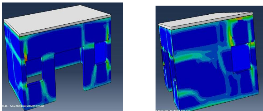
شکل ۷. کانتور کرنش‌های پلاستیک اصلی پیشینه در چهار وجه ساختمان
