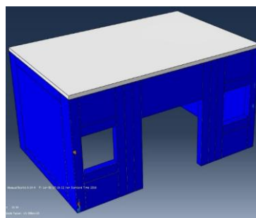
شکل ۱۹. کانتور کرنش‌های پلاستیک اصلی پیشینه بعد از تقویت در مقابل زلزله طیس که در ایستگاه بجستان (خاک نوع II) ثبت شده است
