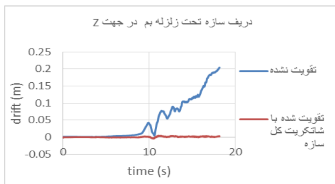
شکل ۱۳. نمودار دررفت سازه تحت زلزله بم
