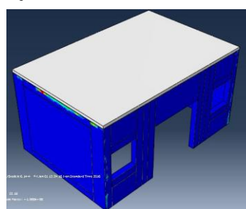
شکل ۱۷. کانتور کرنش‌های پلاستیک اصلی پیشینه بعد از تقویت در مقابل زلزله طبرس که در ایستگاه کاشمر (خاک نوع III) ثبت شده است
