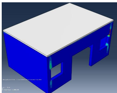
شکل ۱۸. کانتور کرنش‌های پلاستیک اصلی پیشینه قبل از تقویت در مقابل زلزله طبرس که در ایستگاه بجستان (خاک نوع II) ثبت شده است
