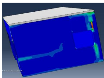
شکل ۱۶. کانتور کرنش‌های پلاستیک اصلی پیشینه قبل از تقویت در مقابل زلزله طبرس که در ایستگاه کاشمر (خاک نوع III) ثبت شده است
