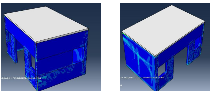
شکل ۸. کانتور کرنش‌های پلاستیک اصلی پیشینه در چهار وجه ساختمان
