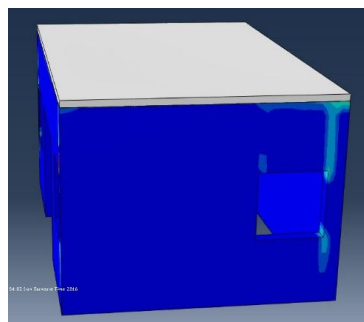
شکل ۱۸. کانتور کرنش‌های پلاستیک اصلی پیشینه قبل از تقویت در مقابل زلزله طبرس که در ایستگاه بجستان (خاک نوع II) ثبت شده است
