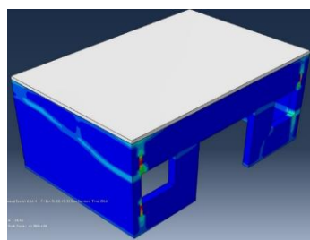
شکل ۱۶. کانتور کرنش‌های پلاستیک اصلی پیشینه قبل از تقویت در مقابل زلزله طبرس که در ایستگاه کاشمر (خاک نوع III) ثبت شده است
