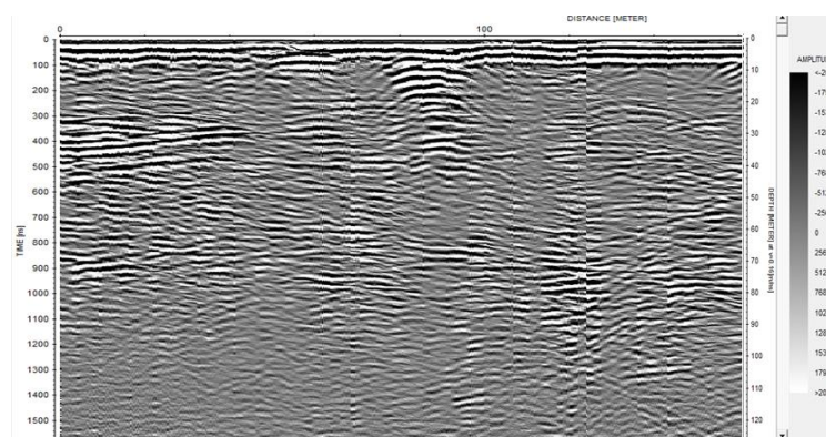
شکل ۵. نگاشت راداری داده‌های GPR بعد از به‌کارگیری بهره‌ی ترکیبی خطی و نمایی
