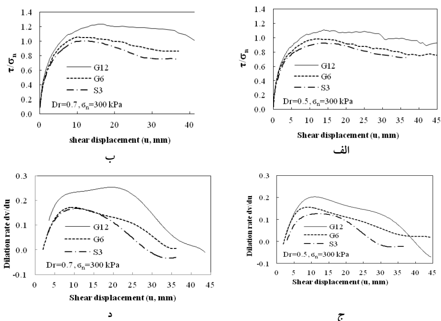
شکل ۵. رفتار برشی و اتساعی برای سه نوع خاک تحت سربار ۳۰۰ کیلوپاسکال با دانسیته نسبی (الف و ج) ۵۰ درصد، ب و د) ۷۰ درصد
