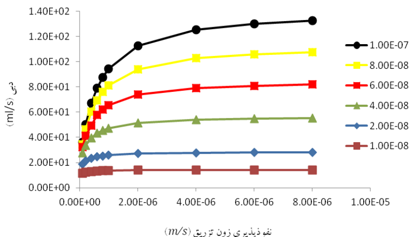
شکل ۸ تأثیر نفوذپذیری پوشش بتنی بر دبی آب ورودی به تونل در پهنه ۷
