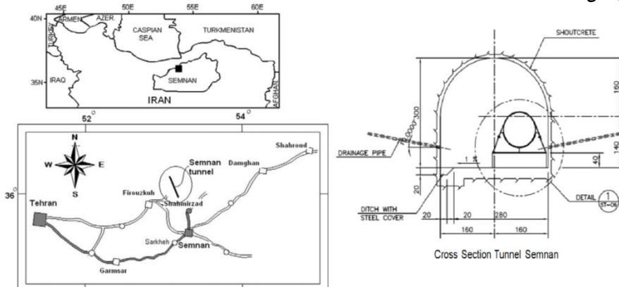
شکل ۱. موقعیت جغرافیایی و مشخصات مقطعی تونل سمنان [۳۳]
