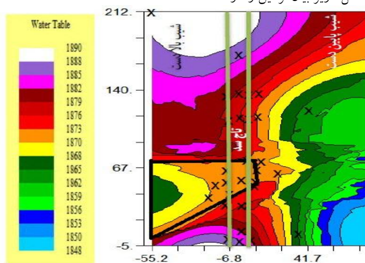
شکل ۵. نقشه دو بعدی هم‌تراز پیزومتریک در بدنه سد جدول ۳. سطح ایستابی آب در پیزومترها نسبت به دریا
