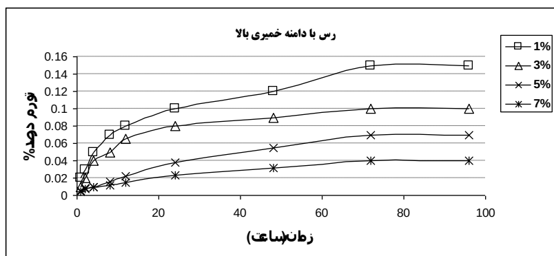
شکل ۱۲. تغییرات درصد تورم با زمان برای درصدهای مختلف افزودنی آهک به خاک رس با دامنه خمیری زیاد
