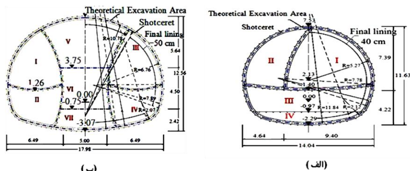
شکل ۳. مقطع عرضی از تونل و مراحل حفاری الف) مسیر دوخطه، ب) مسیر سه‌خطه [۷]
