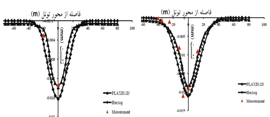
شکل ۱۳. الگوی نشست برای مقطع CS-3
