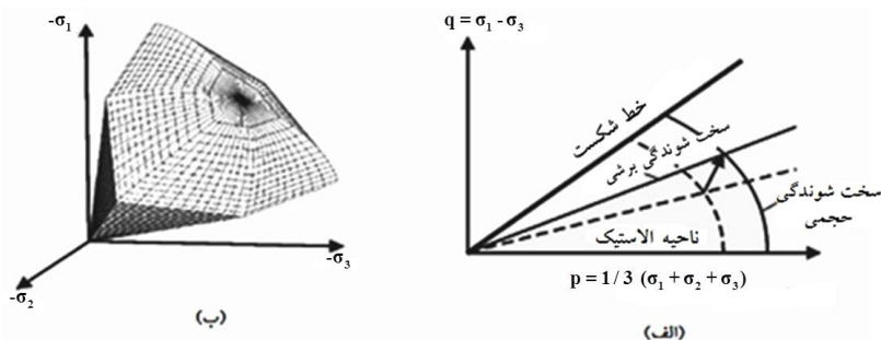
شکل ۶. سطح تسلیم برای مدل خاک سخت‌شونده در C=0 الف) سطح شونددگی برشی و حجمی در فضای p-q ، ب) سطح تسلیم کل در فضای تنش‌های اصلی [۳۱]
