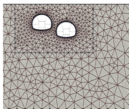
شکل ۱۰. مدل‌بندی المان محدود (کیلومتر ۰+۵۰۵)
