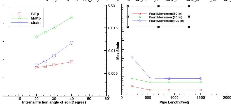
شکل ۶. تغییرات کرنش بیشینه بر حسب جابه‌جایی‌های شکل ۷. پاسخ لوله به حرکات گسل بر حسب زاویه اصطکاک داخلی خاک مختلف گسل در طول لوله
