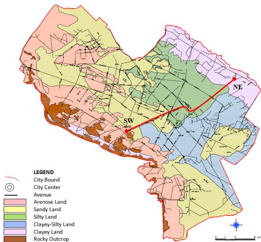
شکل ۱. نقشه پراکندگی سطحی خاک‌های مختلف در بستر شهر مشهد به همراه مسیر خط ۲، [۱].
